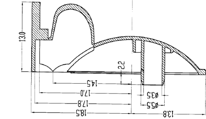
剖面A-A
